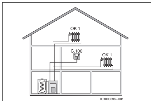
Рис. 1 Пример отопительной системы с одним отопительным контуром НК 1 и C 100 как регулятор (коттедж на одну семью)
