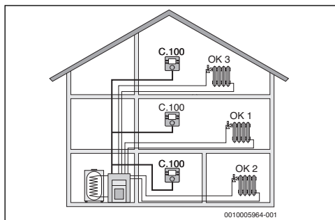
Рис. 3 Пример отопительной системы с тремя отопительными контурами с пультом C 100 как регулятор на каждом (многоквартирный дом)
