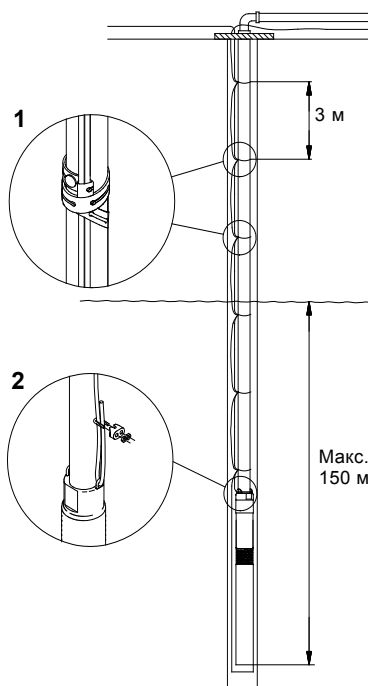
Рис. 18 Подсоединение к трубопроводу
