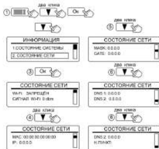
Рисунок 29. Вид вкладки «СОСТОЯНИЕ СЕТИ»
