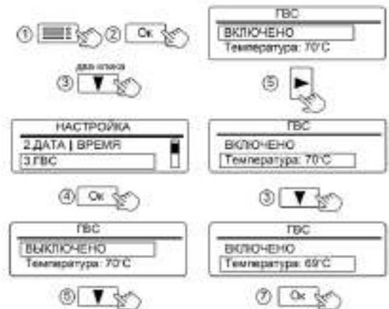
Рисунок 12. Настройка режима «ГВС»
