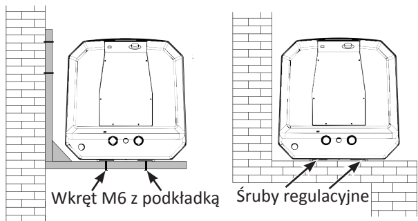
Rys. 4 Poprawny montaż podgrzewacza w pozycji poziomej
