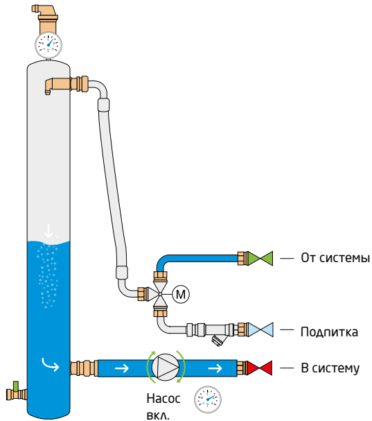
1. Образование вакуума Включение насосов для образования вакуума в трубе.
