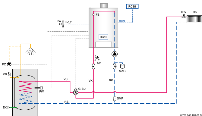
Комплектация котельной с одним контуром отопления и блок косвенного нагрева
