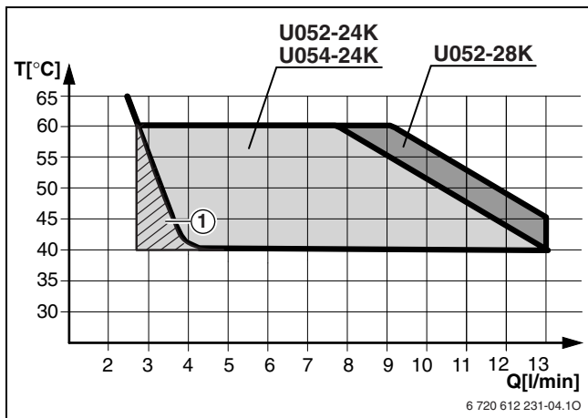
Рис. 9 Диаграмма при температуре холодной воды на входе +15^{\circ}\text{C}
