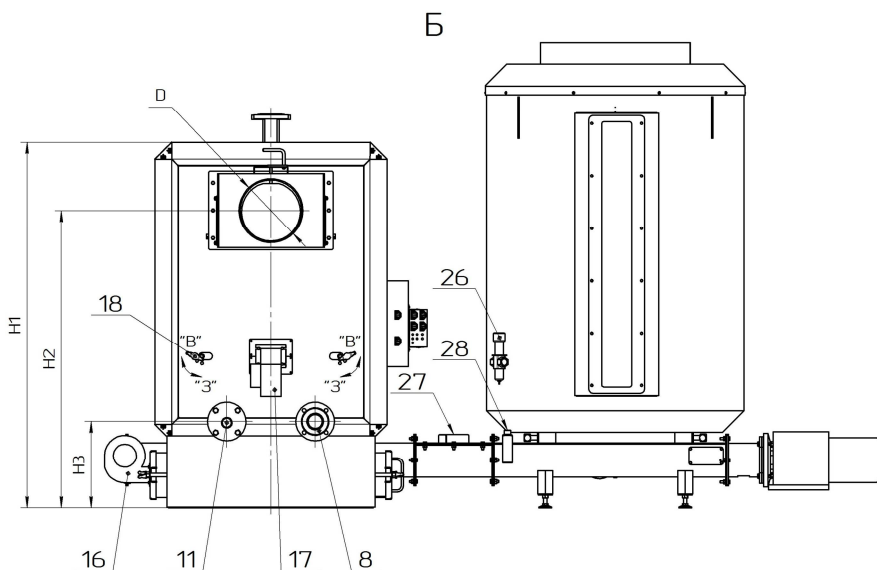
Рисунок 1 - Внешний вид и основные элементы котла
