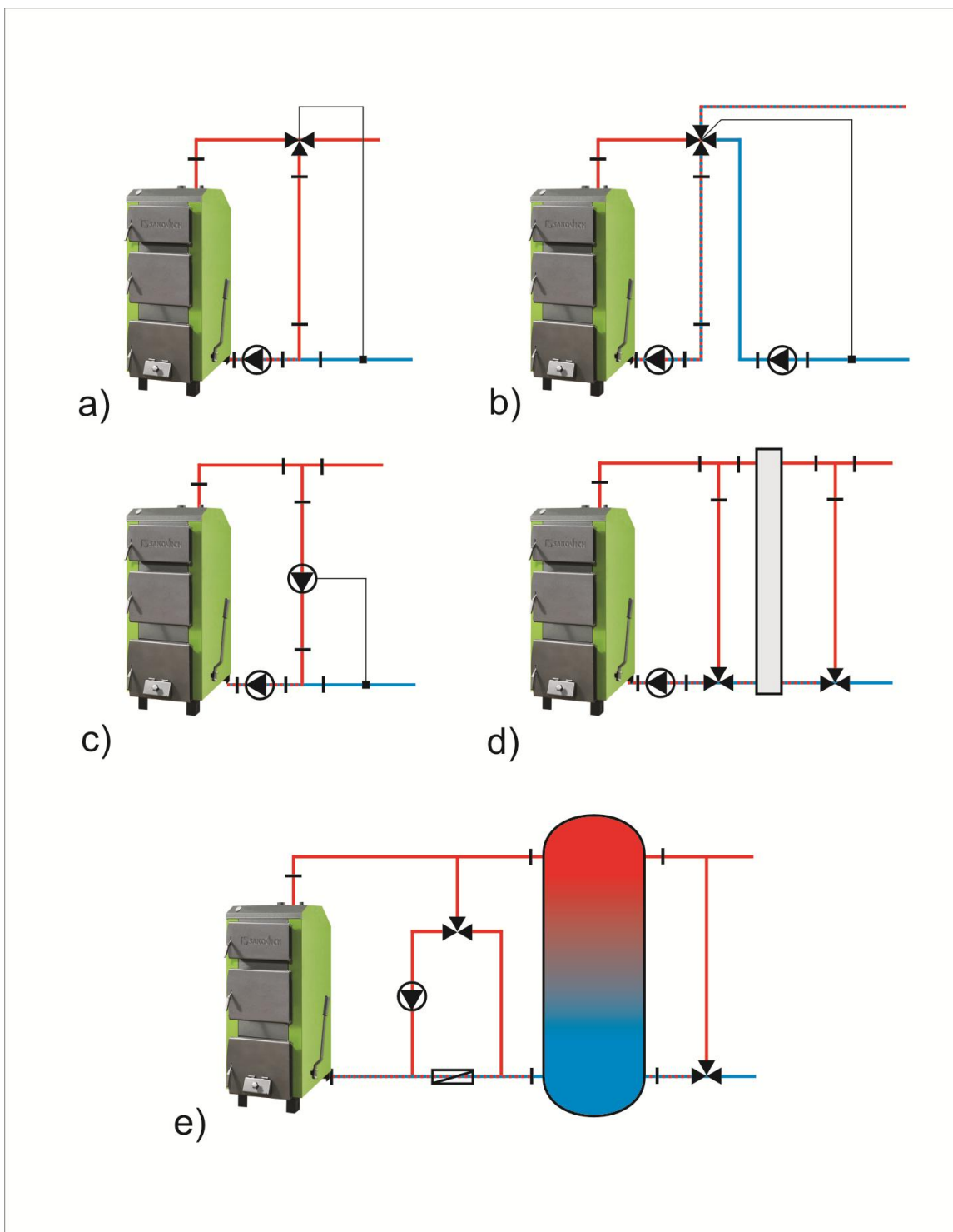
Рис 4. Рекомендуемые схемы соединения котла SAKOVICH Premium с системой отопления: а) с трехходовым клапаном; б) с четырехходовым клапаном; в) с циркуляционным насосом; д) с гидравлической муфтой; е) с буферной ёмкостью
