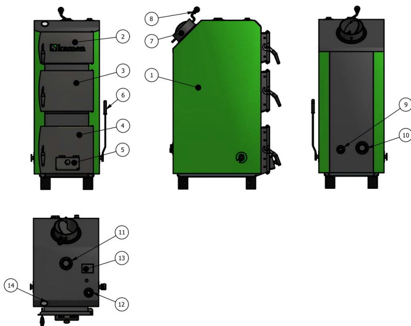
Рис 1. Основные элементы котлов SAKOVICH PREMIUM
