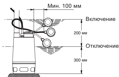
Рис. 7 Уровень вкл./выкл. при мин. длине свободного конца кабеля
