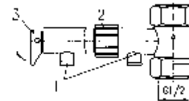
Рис. 4 Предохранительный клапан
