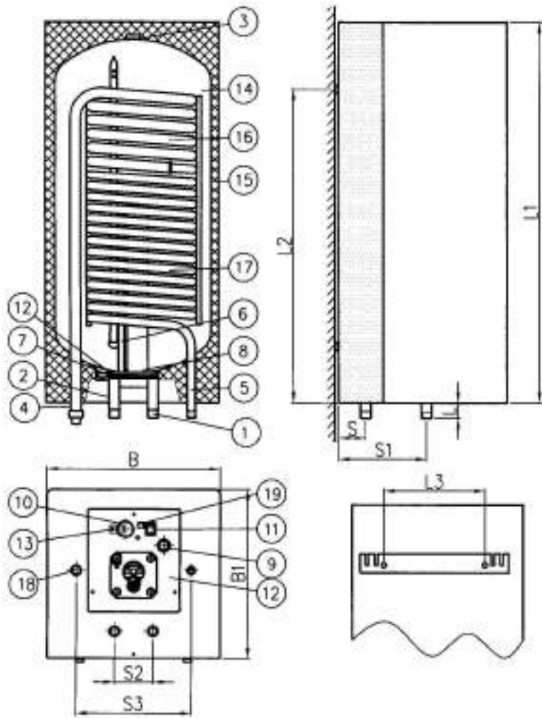
Рис. 1 Конструкция водонагревателя
