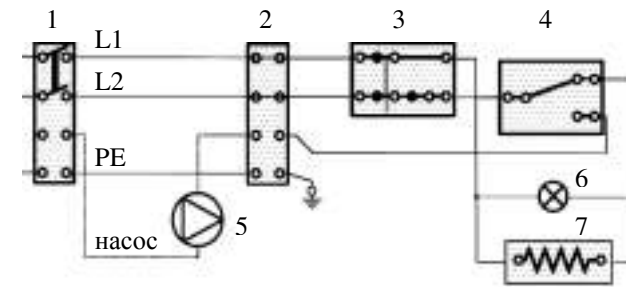
3 Электросхема
