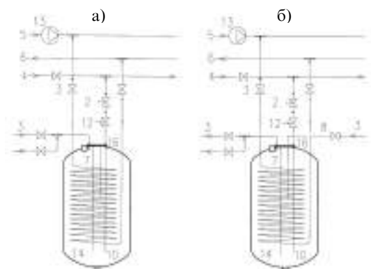
Рис. 5. Схема гидросистемы: а) без циркуляции, б) с циркуляцией 1. воздуховыпускной клапан, 2. редукционный клапан, 3. теплая вода / вход циркуляции, 4. холодная вода, 5. вход теплообменника, 6. выход теплообменника, 7. датчики, 8. циркуляция, 9. водосливной вентиль, 10. эмеевик-теплообменник, 11. ТЭН, 12. предохранительный клапан, 13. циркуляционный насос, 14. трубка РЕХ, 15. тройник, 16. крышка
