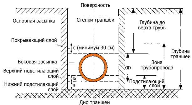
Рис. 3 Устройство траншеи
