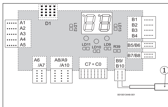
Рис. 1 Подключение датчика к клеммам B9/B10
