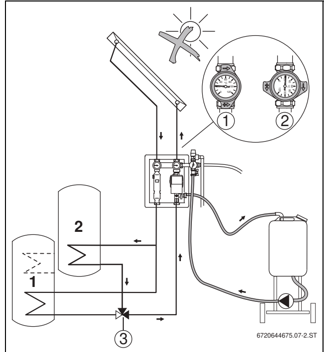
Рис. 29 Промывка бака 2
