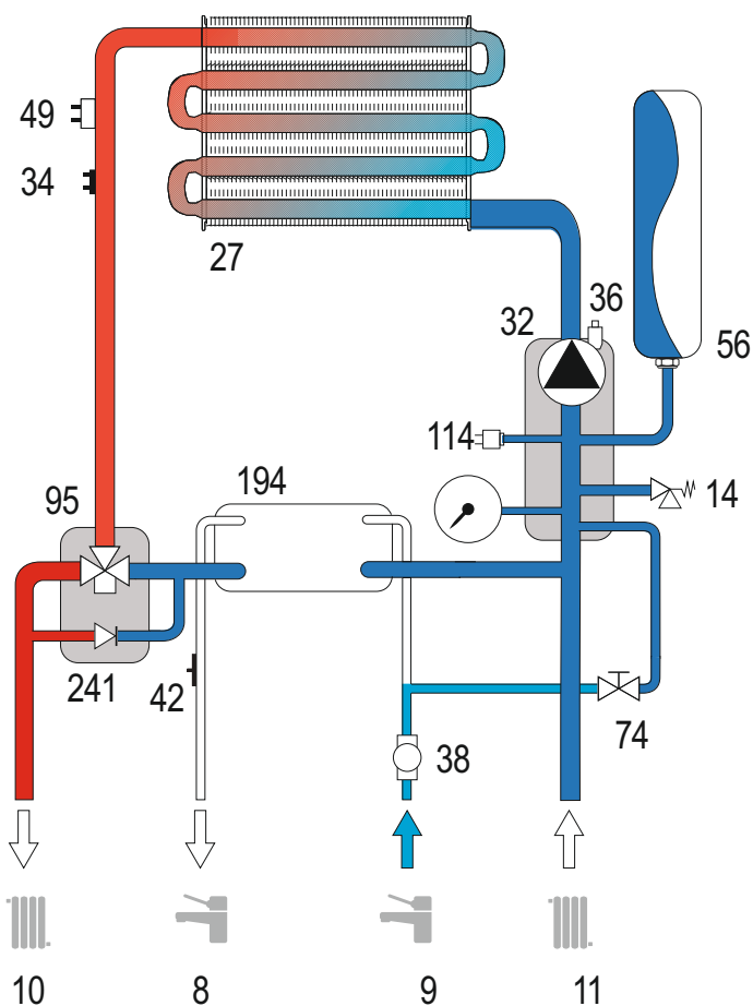
рис. 18 – Контур ГВС
