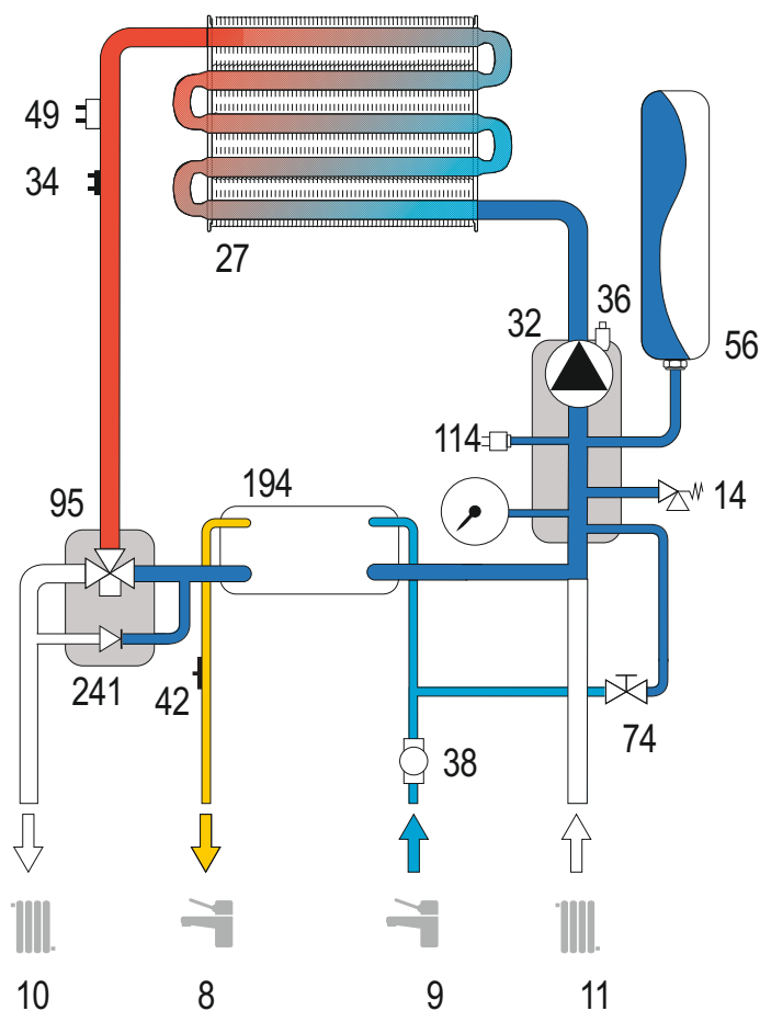
рис. 17 – Отопительный контур
