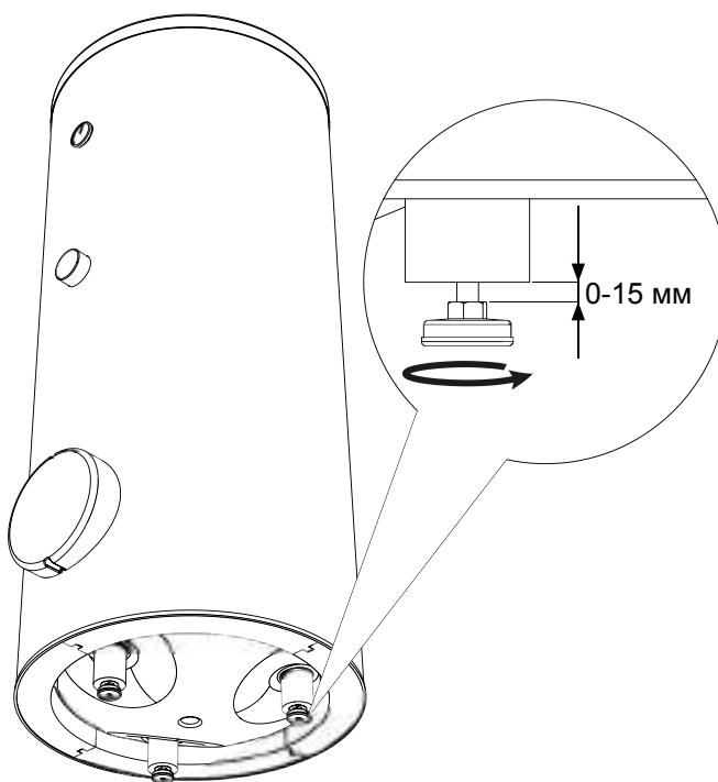
Рис. 10 Выравнивание устройства.
