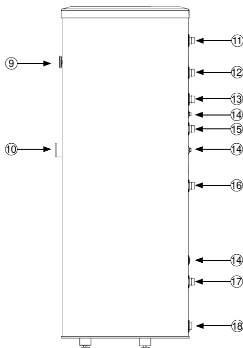
Рис. 3 Вид сбоку водонагревателя W-E 220.82 R
