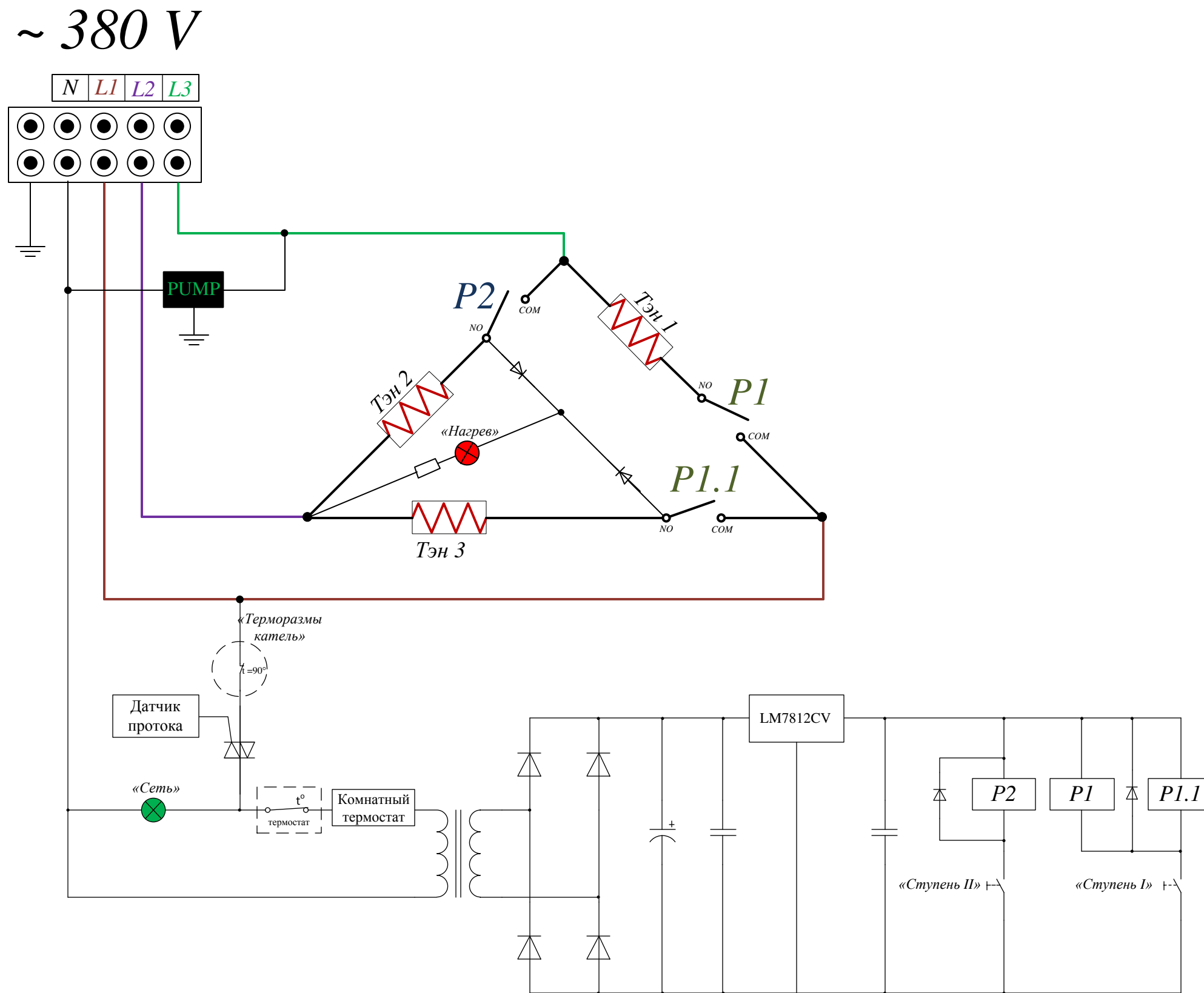
Рисунок 1 – Схема электрическая принципиальная для котлов «Standart» 12, 15 кВт на 380 В
