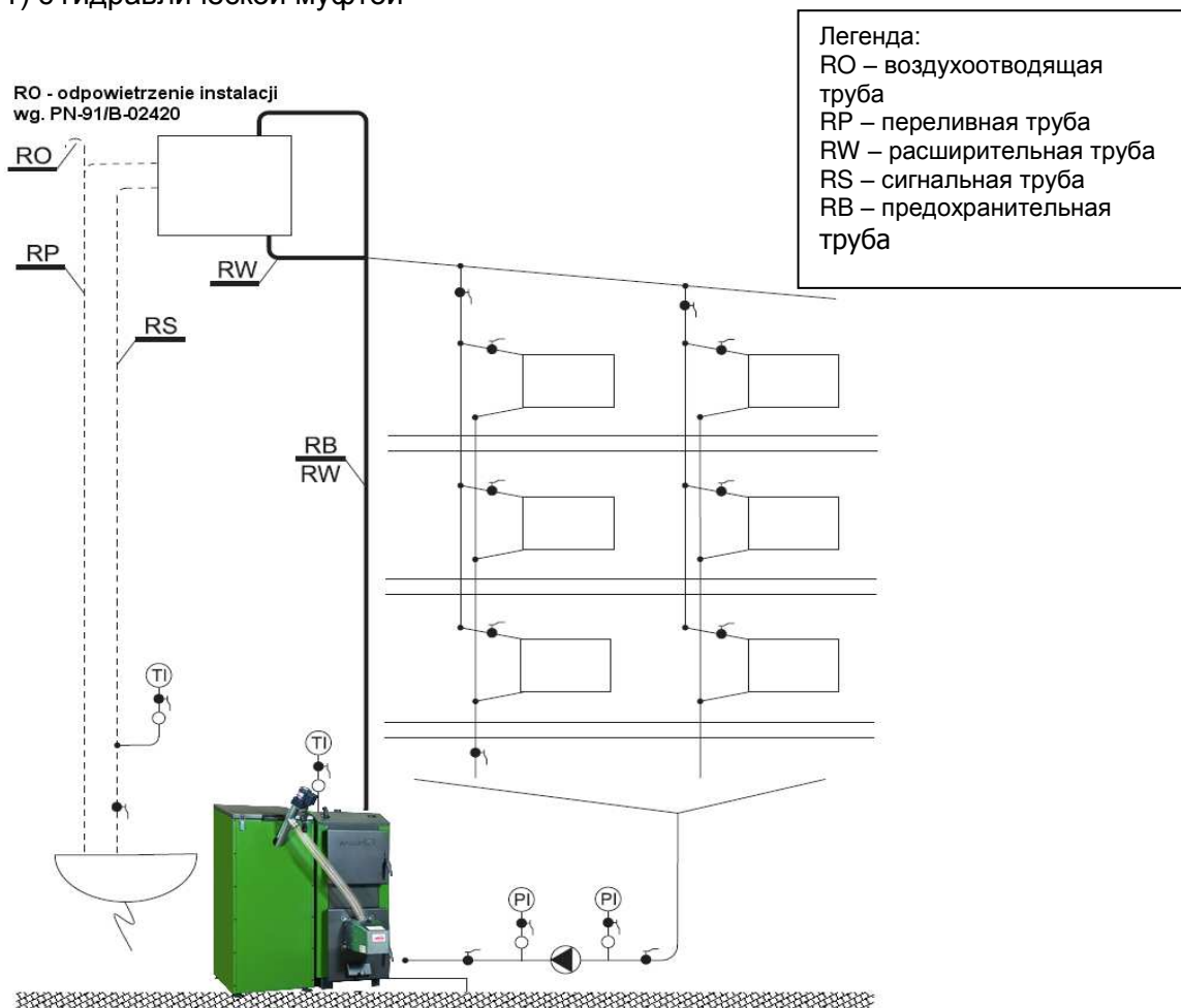
Рис. 4. Рекомендуемые схемы подключения котла SAKOVICH к отопительной системе: а) с трехходовым клапаном; б) с четырехходовым клапаном; в) с циркулярным насосом; г) с гидравлической муфтой
