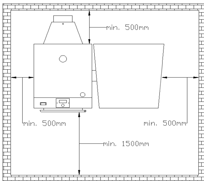
Рис. 3. Установка котла SAKOVICH в помещении котельной.
