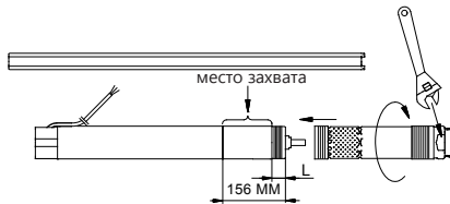
Рис. 13 Затяжка насоса
