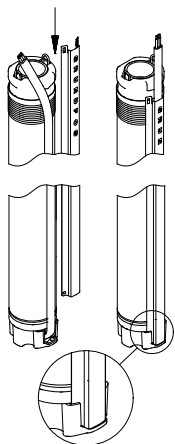
Рис. 16 Установка защитной планки кабеля
