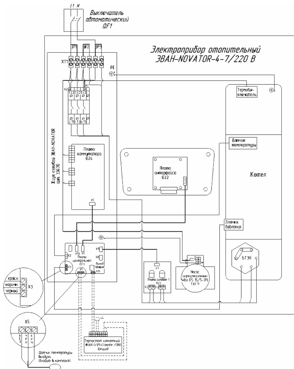
Рисунок 6 Схема подключения ЭВАН NOVATOR -4/7/ 220 В
