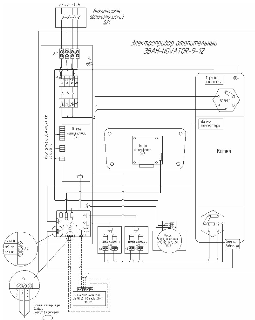
Рисунок 8 Схема подключения ЗБАН NOVATOR -9-12
