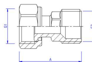
VTr. 613 Соединитель с накидной гайкой В-Н
