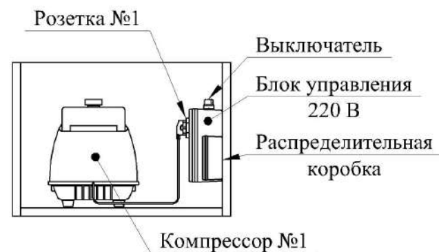
Рис. №1. УОСВ ТОПАС-С 4 -12 с самотечным отводом очищенной воды
