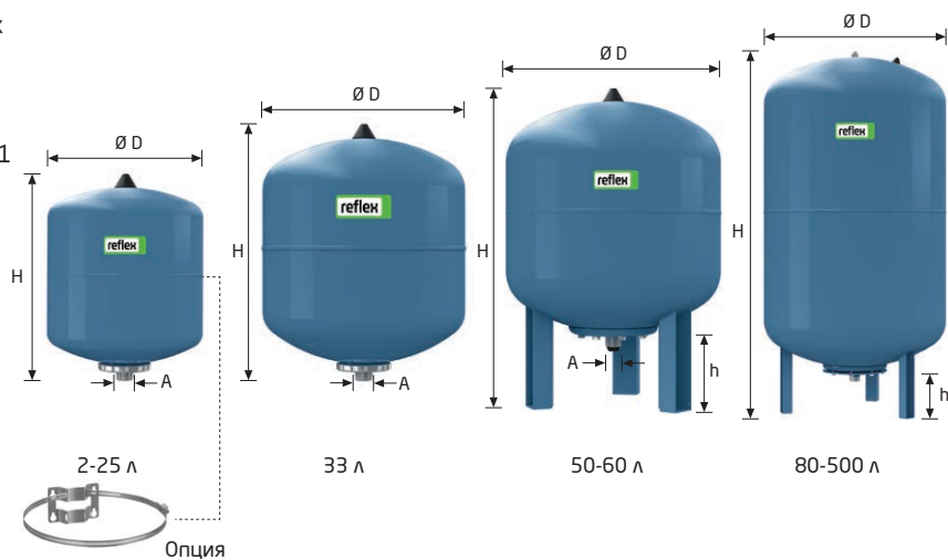
Опция Ленточный хомут для крепления на стене Артикул № 7611000
