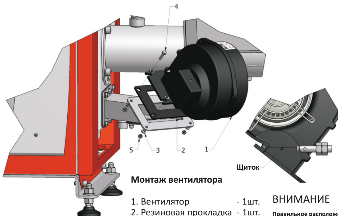
Рис.17 Установка вентилятора
