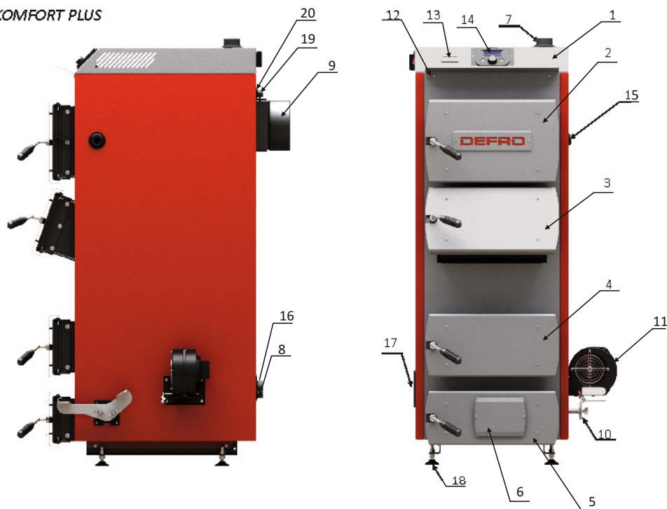
Рис.4. Основные элементы котлов типа NOWA OPTIMA KOMFORT PLUS с оснащением:
