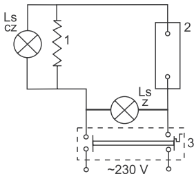
Электрическая схема 230 V~ (Нагревательный элемент 2-3 кВт)
