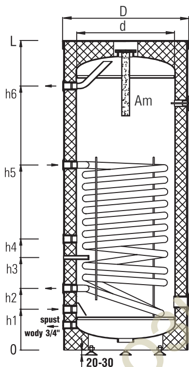
Водонагреватель SGW(S) 100÷140 л
