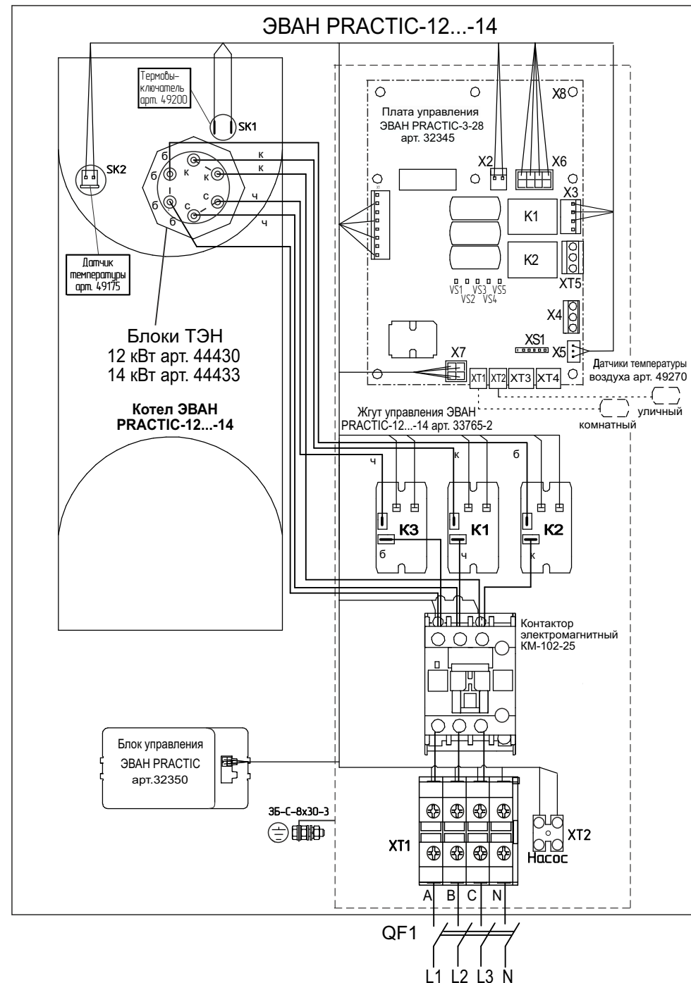
Рисунок 20. Схема подключения ЭВАН PRACTIC-12...-14.
