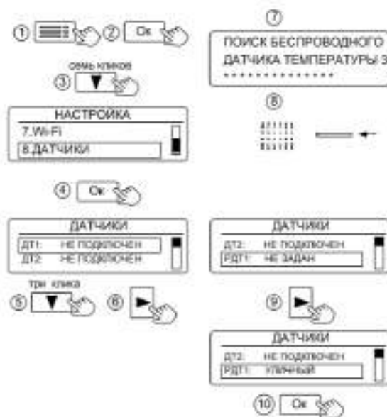
Рисунок 23. Настройка радиодатчиков
