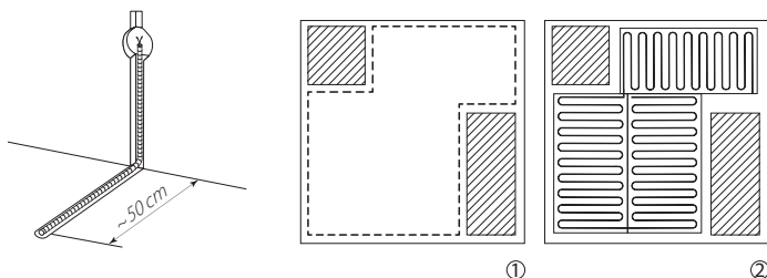
Рисунок 3. 1. Определение площади обогрева. 2. Нагревательный мат после укладки.
