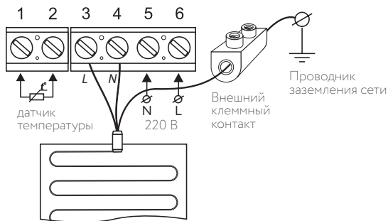
Рисунок 8. Схема подключения мата к сети (220 В)
