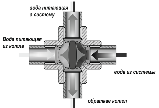
в) Частично открытая система - питающая воды из котле смешивается с водой в системе отопления.
