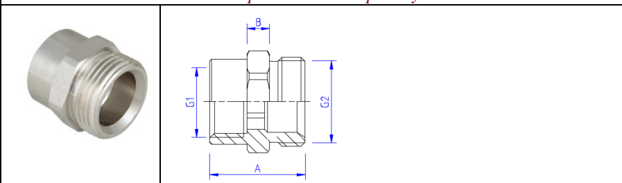
VTr. 592 NE Соединитель с переходом на «еврокonus» В-Н
