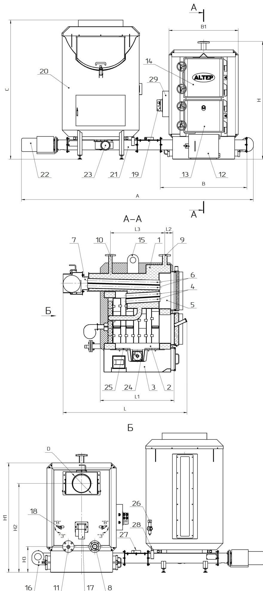
Рисунок 1 - Внешний вид и основные элементы котла
