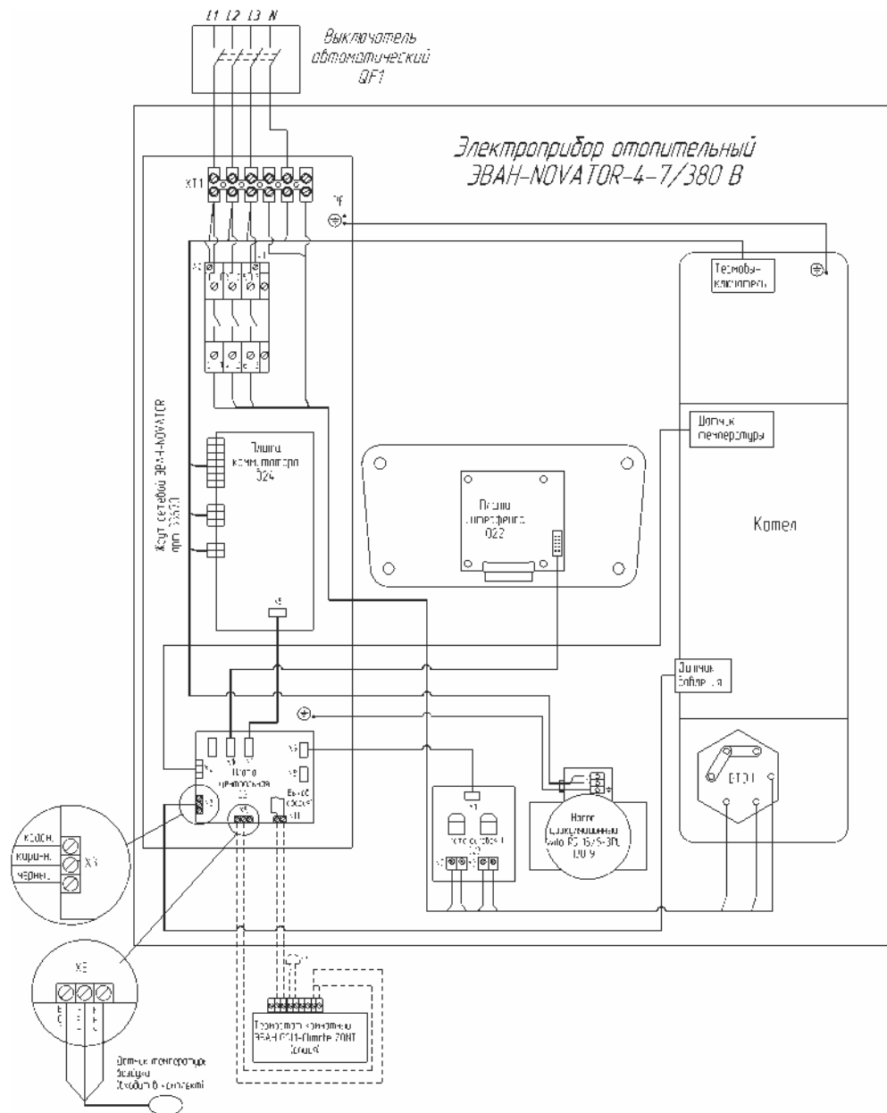
Рисунок 7 Схема подключения ЭВАН NOVATOR -4-7/380 В
