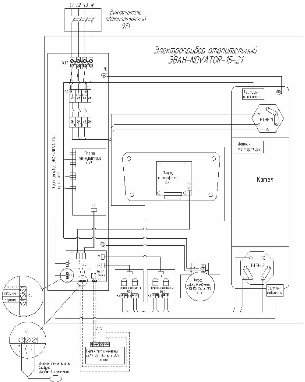
Рисунок 9 Схема подключения ЭВАН NOVATOR -15-21
