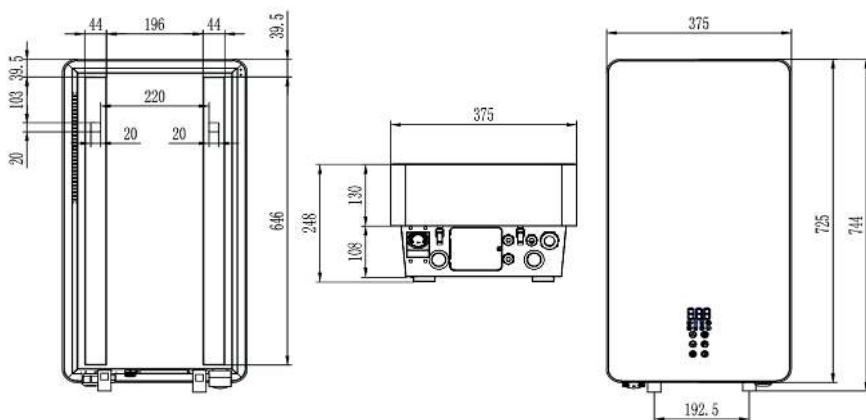
Рисунок 6 - Основные размеры
