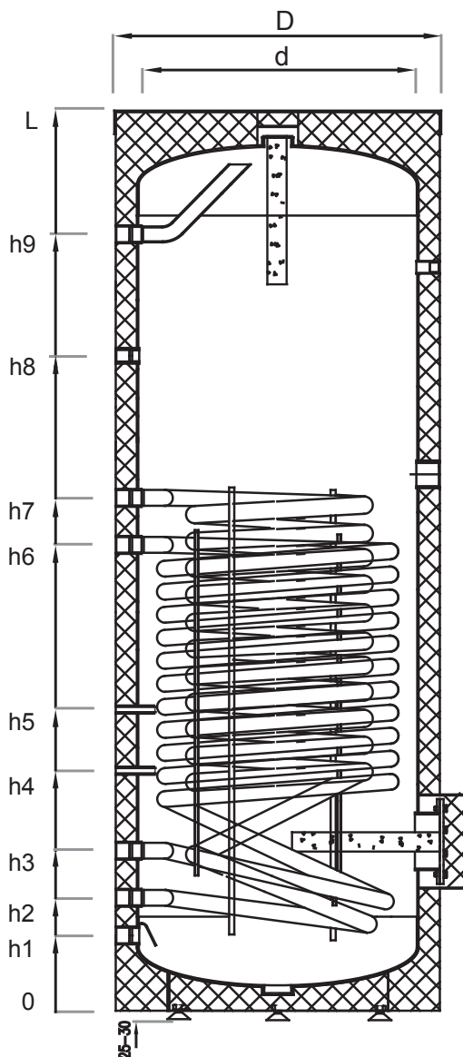
Водонагреватель SGW(S)B 300-500 с двумя теплообменниками в нижней части бака
