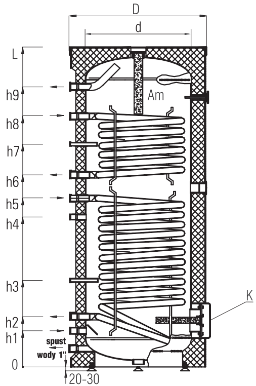
Водонагреватель SGW(S)B 250÷1500 л
