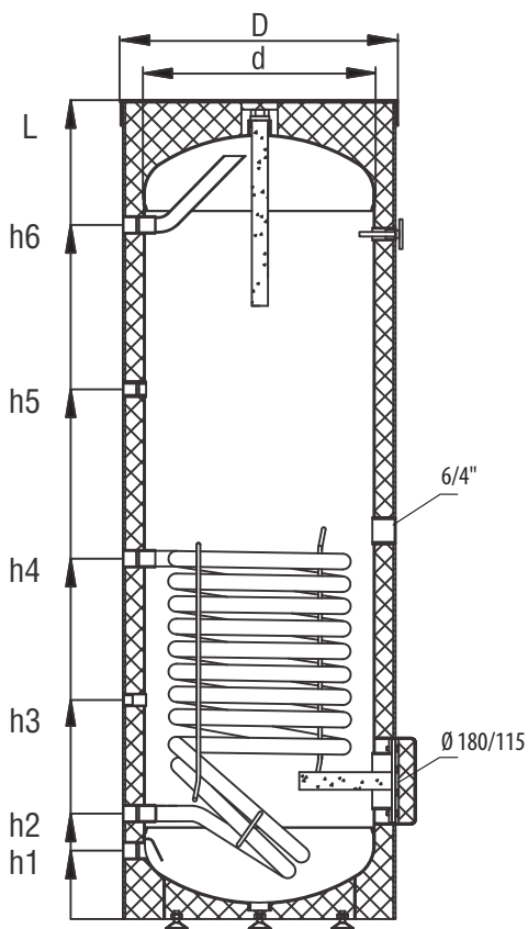
Водонагреватель SGW(S) SLIM 250÷300 л
