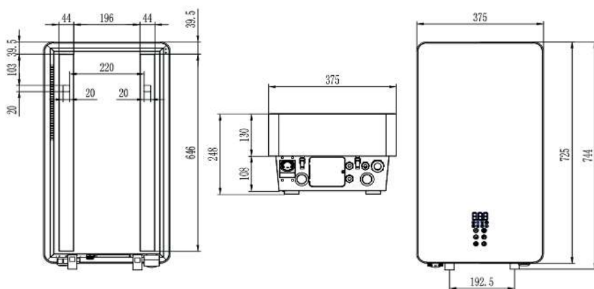
Рисунок 6 - Основные размеры
