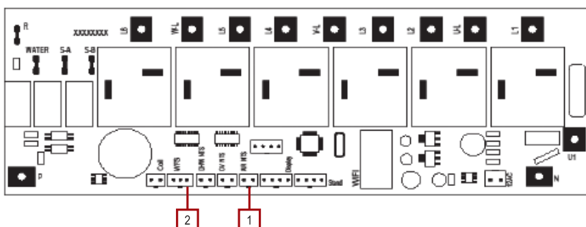
Рисунок 17 - Плата котла
