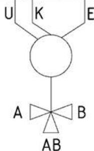
Рисунок 24 - Электроподключение привода трехходового клапана
