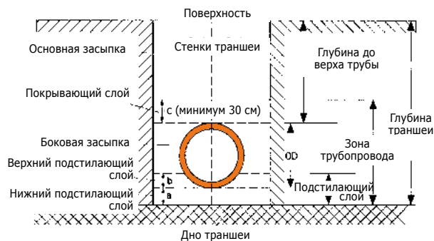
Рис. 3 Устройство траншеи
